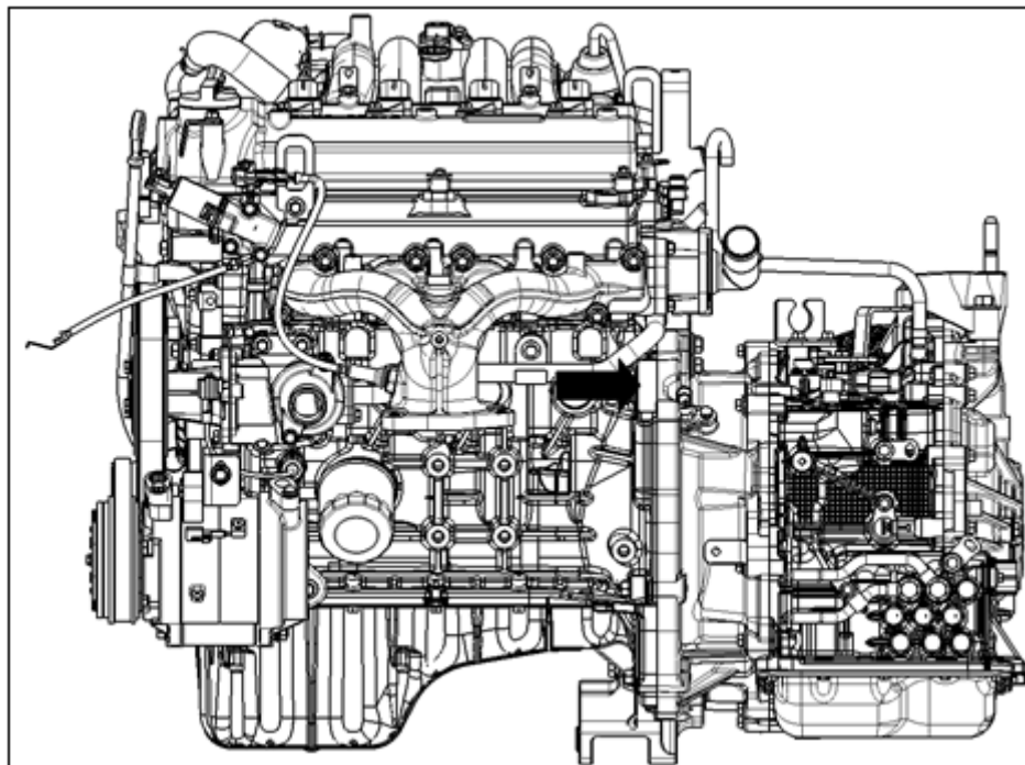
Motor SFG15A+CVT
