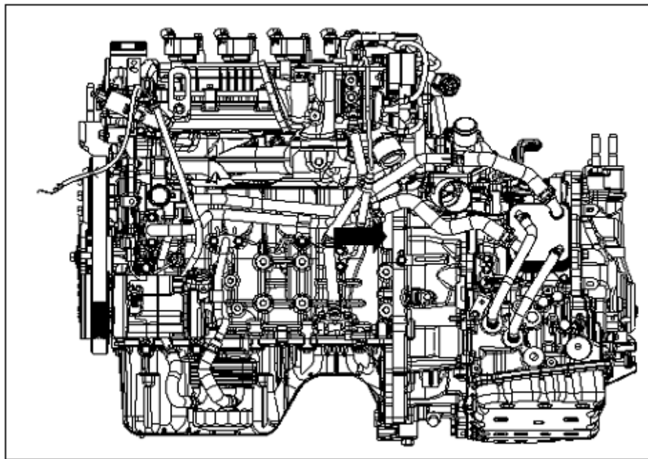
Motor SFG15TA+CVT
