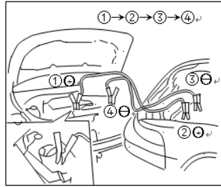
Esquema de arranque del motor por otra batería
