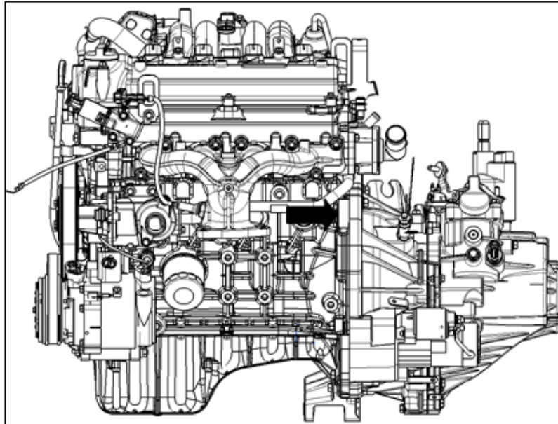
Motor SFG15A+5MT
